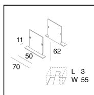
100650.01 End caps (2pcs.)
