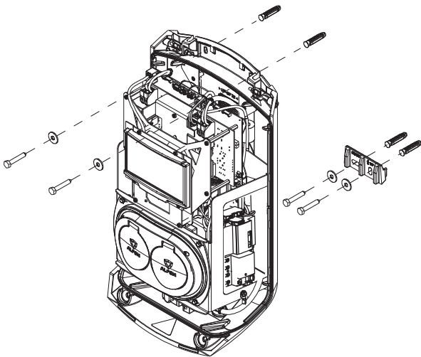
Afbeelding 3: Wandmontage
