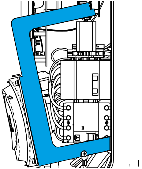
Afbeelding 5: Afneembaar subframe
