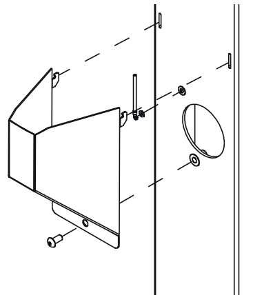
Afbeelding 4: De kabelafdekking vastmaken
